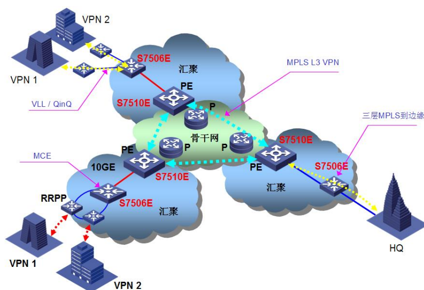
图 2 H3C S7500E 在 MPLS 组网中的典型应用
