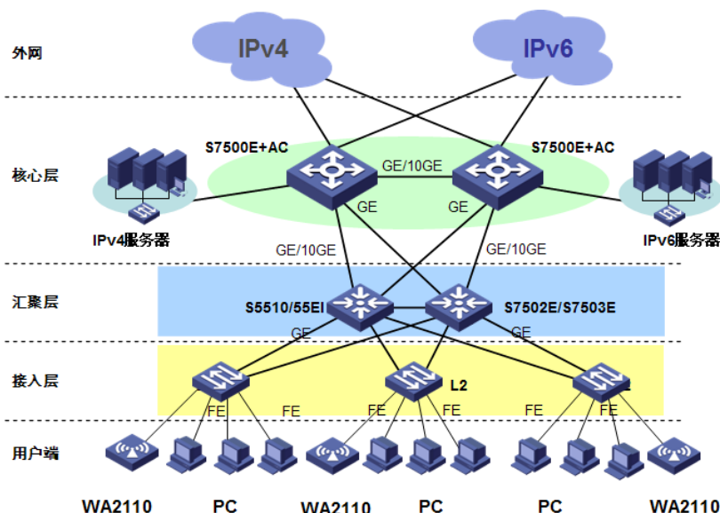
图 3 H3C S7500E 在 Ipv6 校园网典型应用
